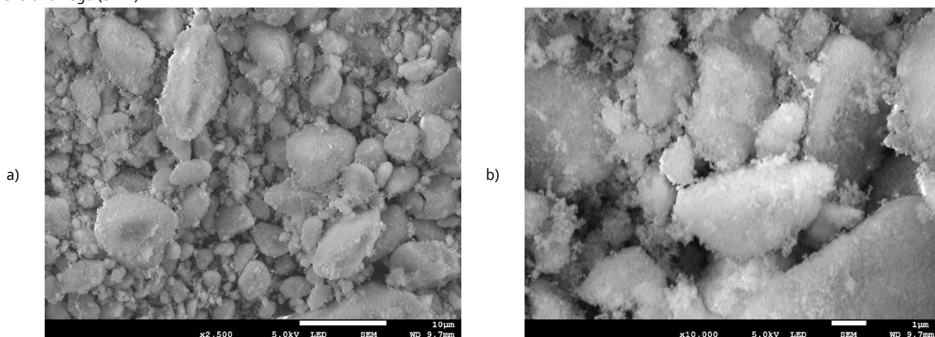
Rys. 1. Zdjęcia ze skaningowego mikroskopu elektronowego dodatku POLYDEF Ag a) powiększenie 2 500 razy, b) powiększenie 10 000 razy
