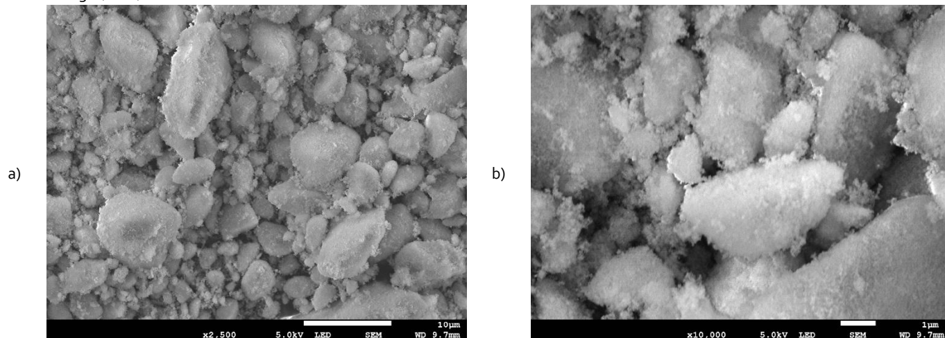
Rys. 1. Zdjęcia ze skaningowego mikroskopu elektronowego dodatku POLYDEF Ag a) powiększenie 2 500 razy, b) powiększenie 10 000 razy
